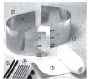
鉄製半割継手 (φ1100~φ1500)
