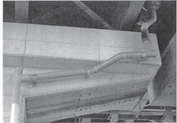
塩ビ管 施工例
