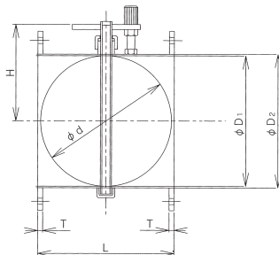
フランジ式 丸ダンパー(1000φ~1500φ)
