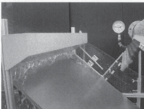
鉄・アルミ板のエアブロー
