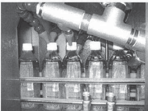
ビン・缶類のエアブロー
