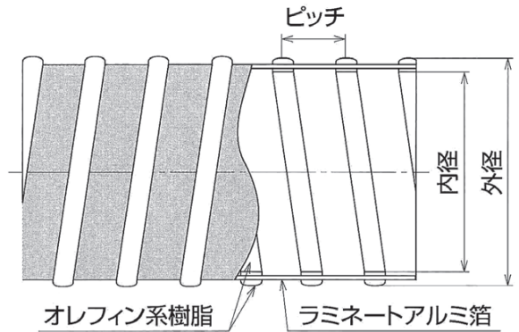
構造図
